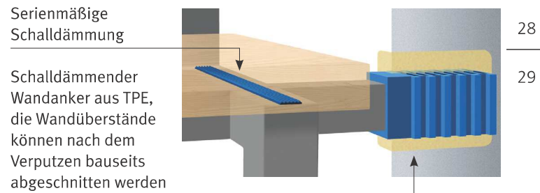
Serienmäßige Schalldämmung, gestemmt
