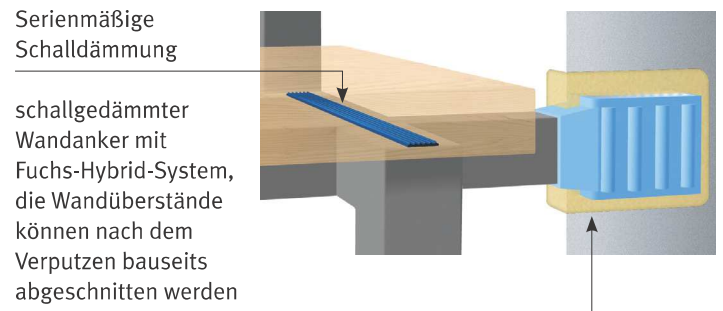
Optional: Erhöhte patentierte Schalldämmung, gestemmt
