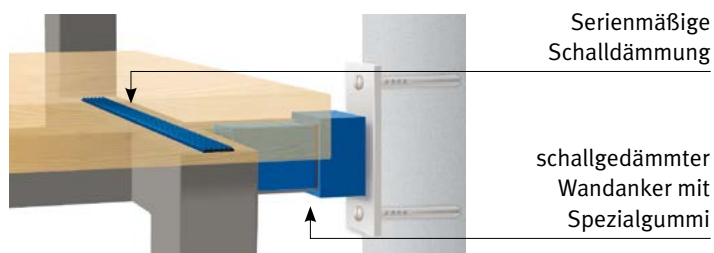
Serienmäßige Schalldämmung, schraubbar
