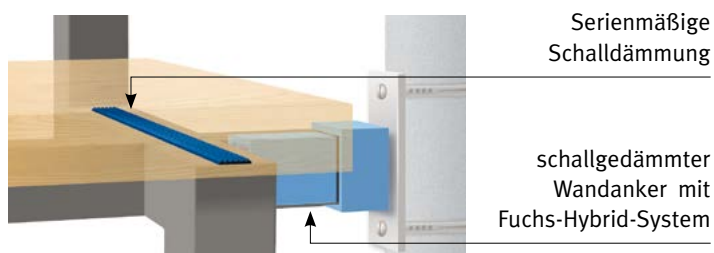
Optional: Erhöhte Schalldämmung, schraubbar
