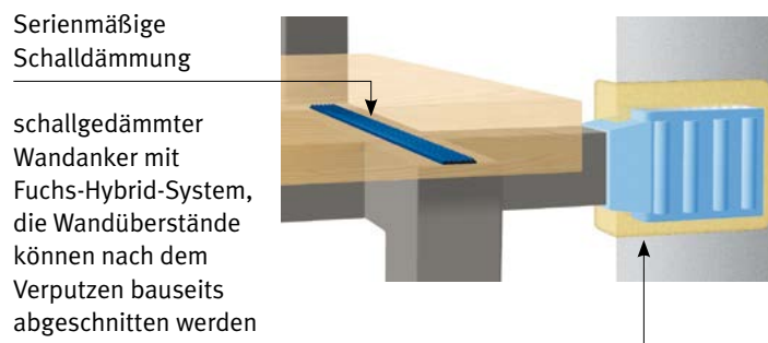
Optional: Erhöhte patentierte Schalldämmung, gestemmt
